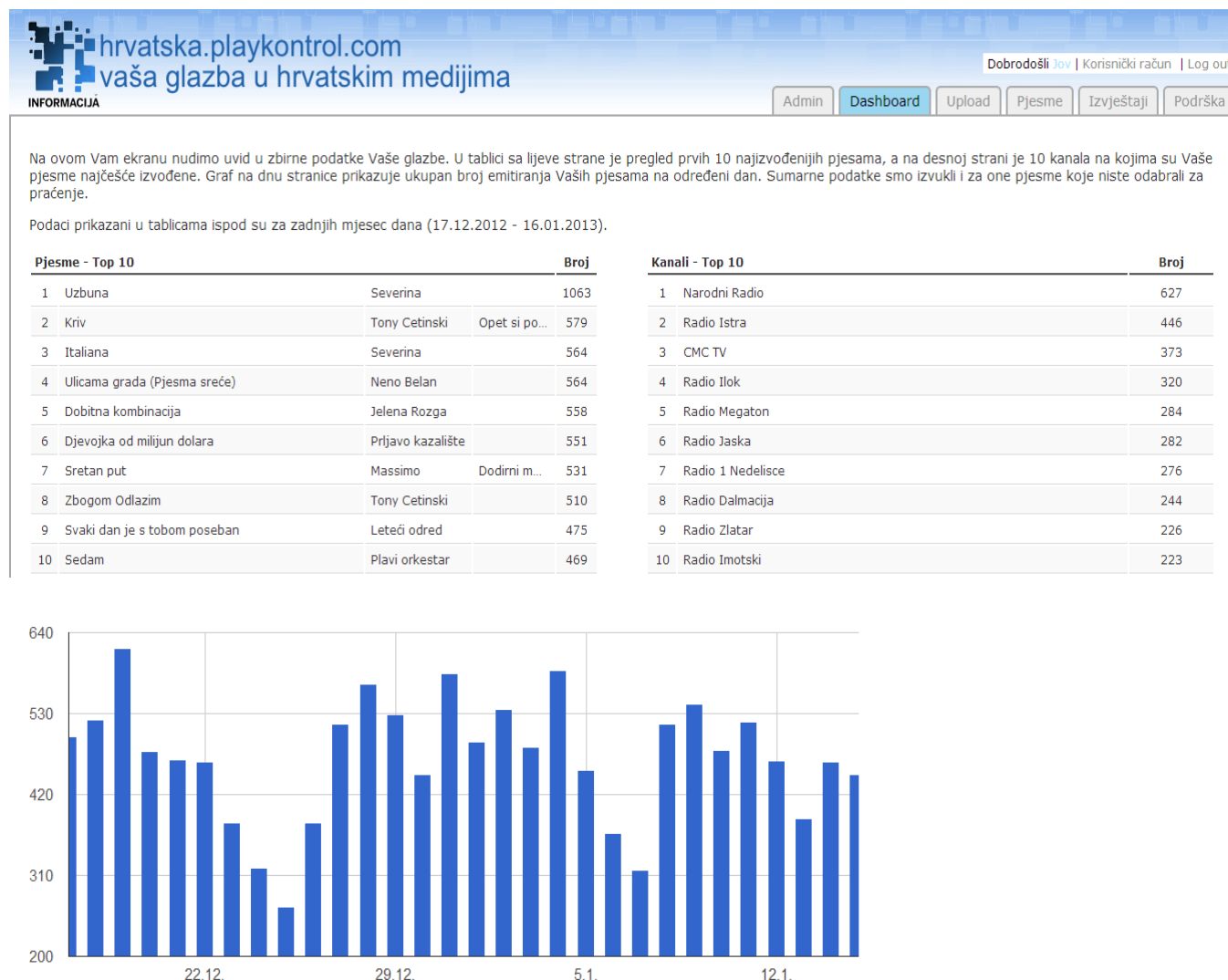
Slika 5 (dashboard stranica)
