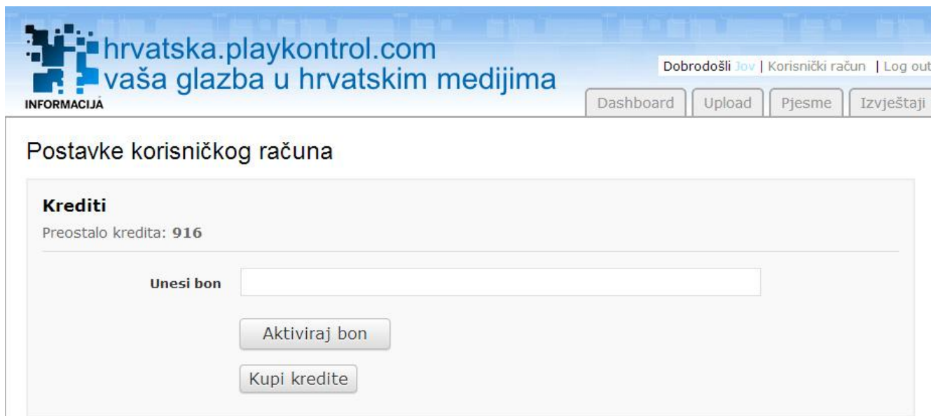
Slika 7 (kupnja kredita)
